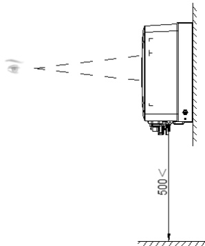
图 4.3 最佳安装高度区域
