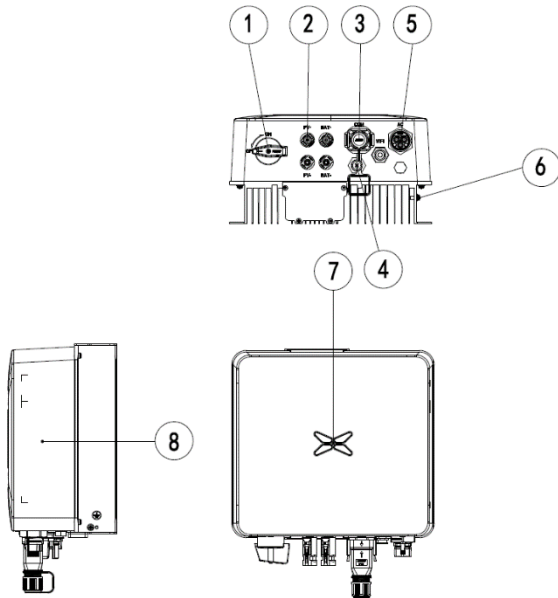
图 2.2 单相光伏逆变器外观图
