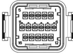
图 5.7 DRM &amp; CT 端子正视图
