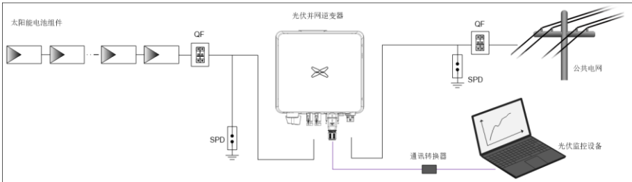
图 5.1 光伏并网系统连接示意图
