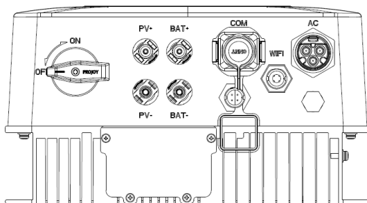
图 2.8 XG1-5KTL-S 底部视图
