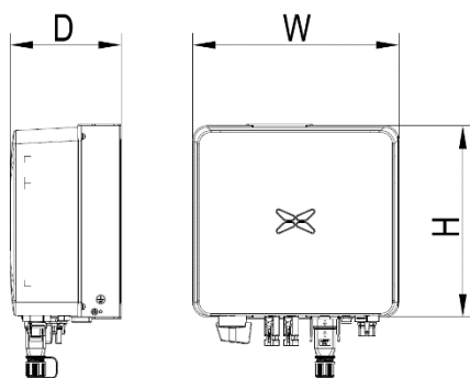
图 2.4 逆变器外形尺寸
