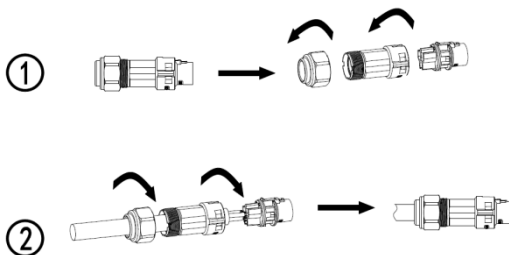
图 5.8 压接电缆端子
