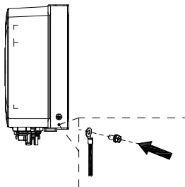
图 5.2 光伏接地示意图
