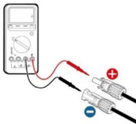
图 5.4 测量直流输入电压
