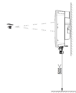
图 4.3 最佳安装高度区域
