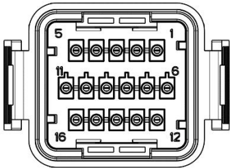
图 5.7 DRM & CT 端子正视图
