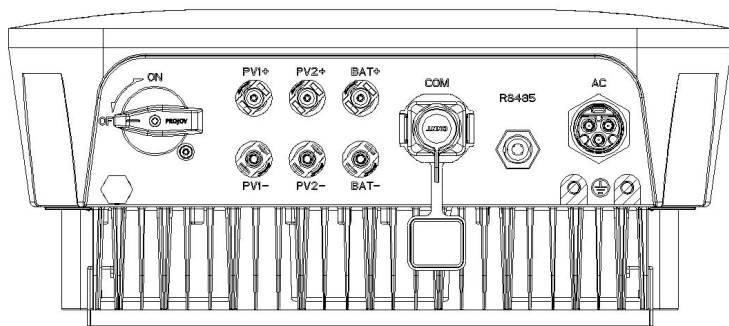
图 2.9 不带风扇
