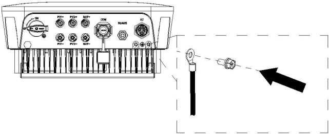
图 5.2 光伏接地示意图
