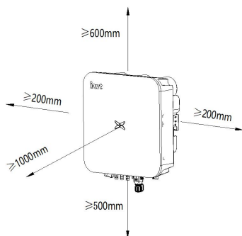
图 4.4 逆变器安装间距
