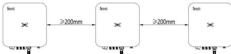
图 4.5 并排安装尺寸要求
