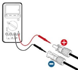
图 5.4 测量直流输入电压
