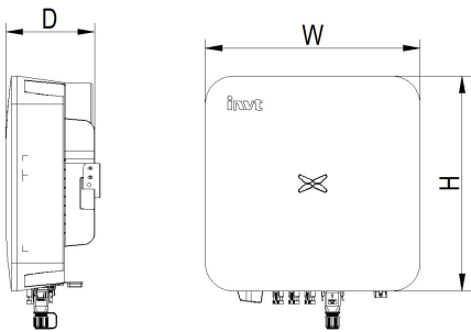
图 2.5 逆变器外形尺寸
