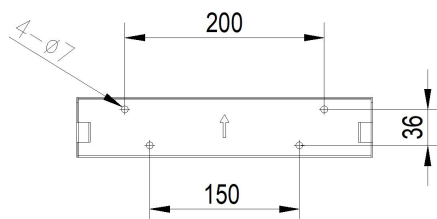
图 4.6 安装挂板尺寸图
