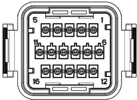
图 5.7DRM &CT 端子正视图
