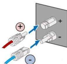
图 5.5 光伏直流组串接入逆变器
