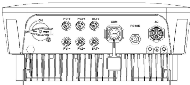
图 2.9 不带风扇
