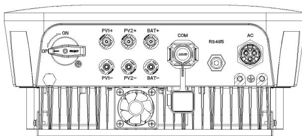
图 2.10 带风扇 (XG7KTL1/ XG8KTL1/ XG10KTL/ XG10KTL1)
