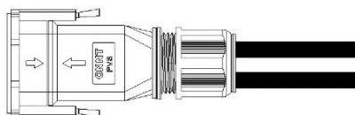
图 5.6 DRM &CT 端子侧视图
