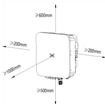
图 4.4 逆变器安装间距
