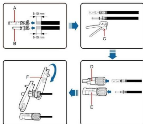
图 5.3 MC4 直流连接器与光伏组串的连接
