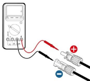
图 5.4 测量直流输入电压
