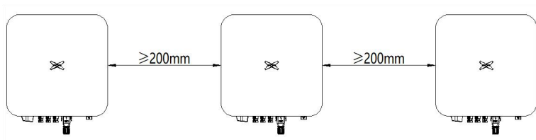
图 4.5 并排安装尺寸要求
