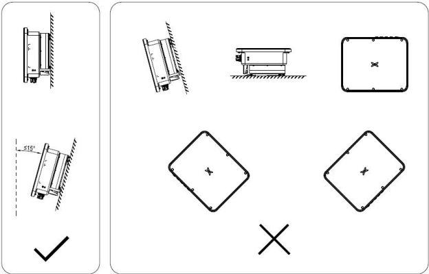
图 4.6 逆变器安装位置
