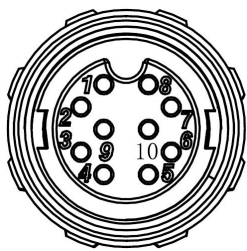
图 5.7 DRM & RS485 端子正视图
