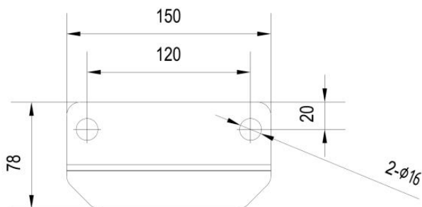
图 4.7 安装挂板尺寸图
