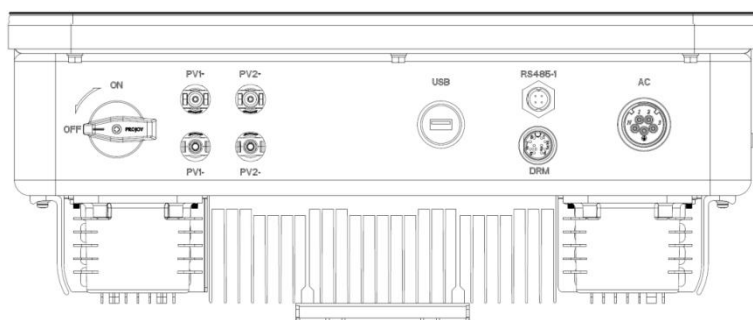
图 2.10 XG3-12KTR 底部视图
