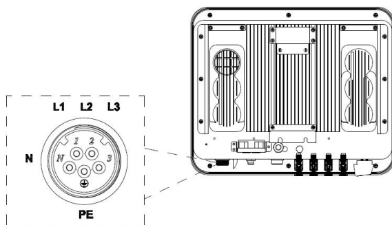
图 5.9 三相逆变器电网接入
