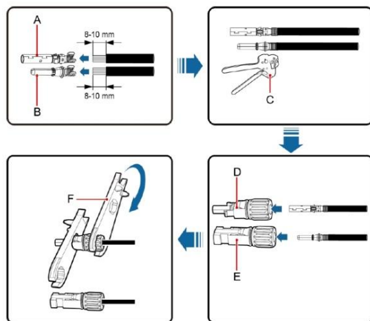
图 5.3 MC4 直流连接器与光伏组串的连接
