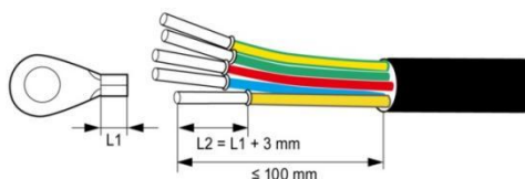
图 5.8 压接电缆端子
