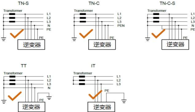
图 2.2 光伏并网逆变器支持的电网形式
