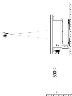
图 4.3 最佳安装高度区域
