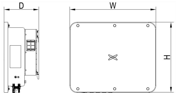
图 2.5 逆变器外形尺寸
